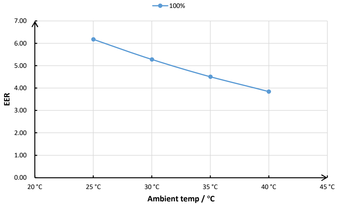
X20-18C EER Curve
